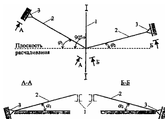
Рисунок Л.2 – Схема раскрепления ферм расчалками
